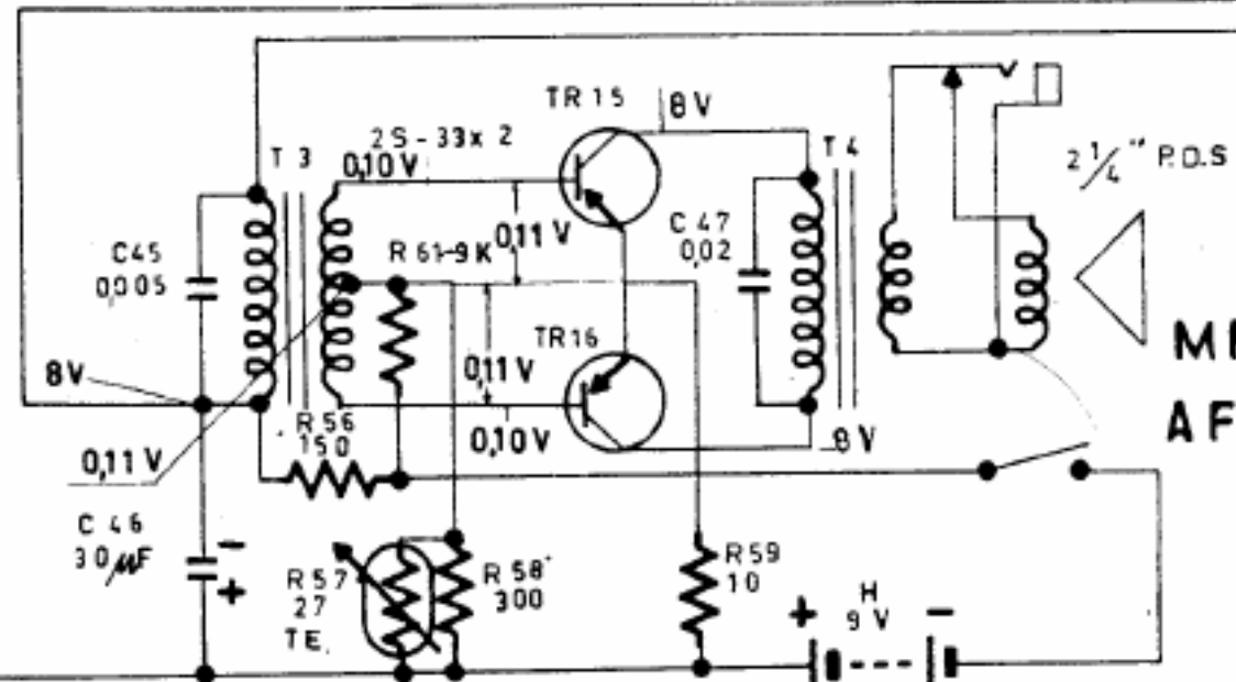
TENSIONI MISURATE CON VOLMETRO WESTON 20000 Ω/V
